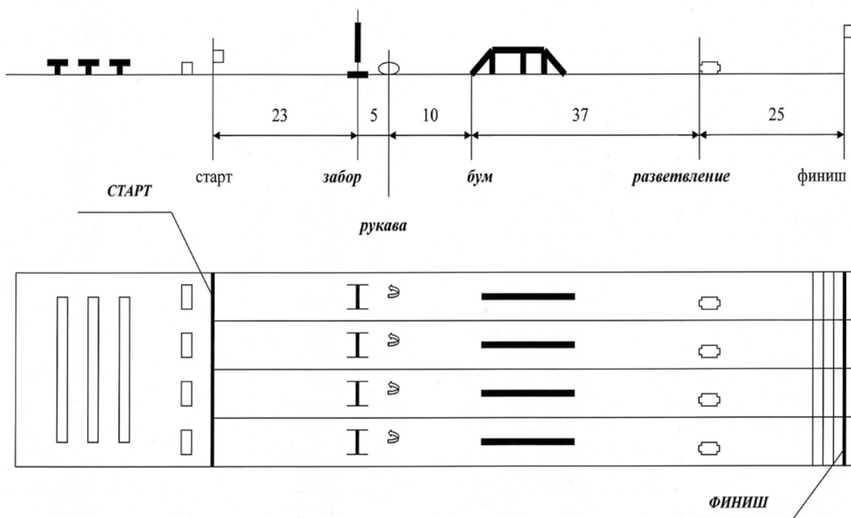
Схема площадки для полосы препятствий
